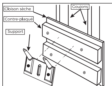
Figure - Montage pour cloison sèche
