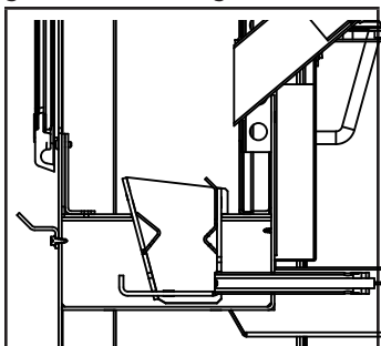
Figure 3 Pot de combustion PS60W et PS130W
