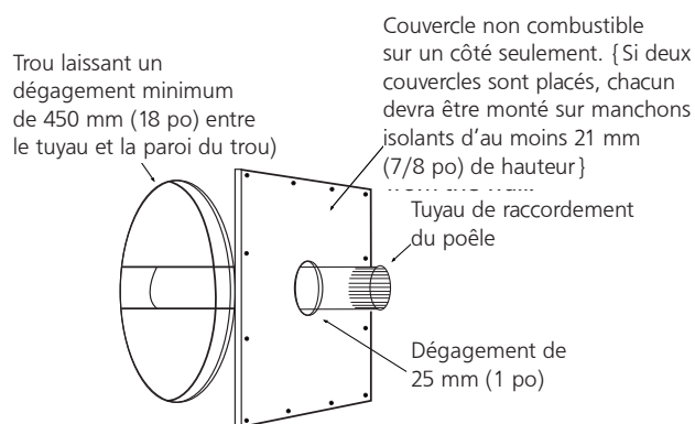
Figure 6 SEULEMENT UN TUYAU DE TRAVERSÉE CONFORME AUX NORMES CANADIENNES
