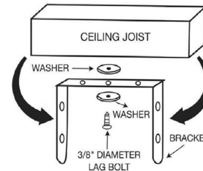
Figure 4a : Montage avec une vis, pour permettre un pivotement
