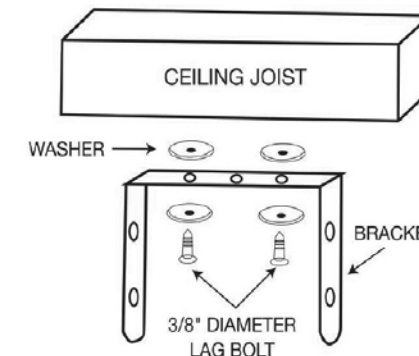
Figure 4b : Montage avec deux vis, pour position fixe
