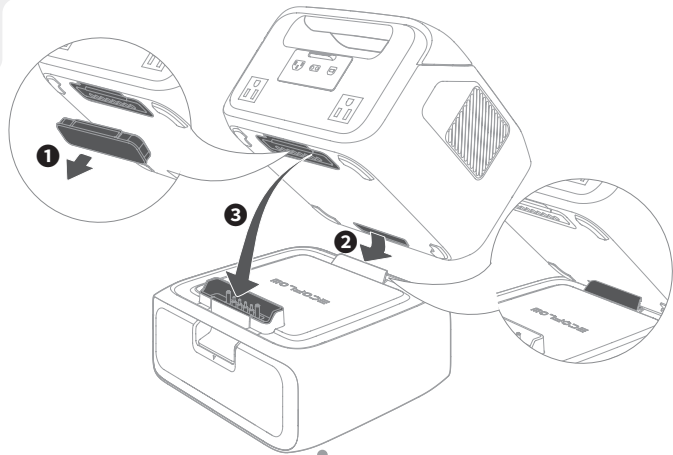
EcoFlow RIVER 3 Plus Smart Extra Battery Batterie supplémentaire intelligente pour EcoFlow RIVER 3 Plus
