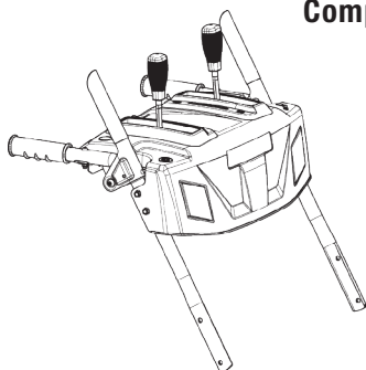
Ensemble de poignée supérieure X 1
