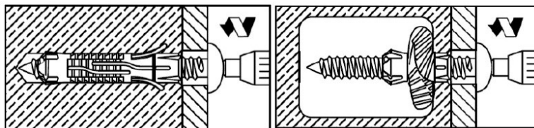
Mur plein
