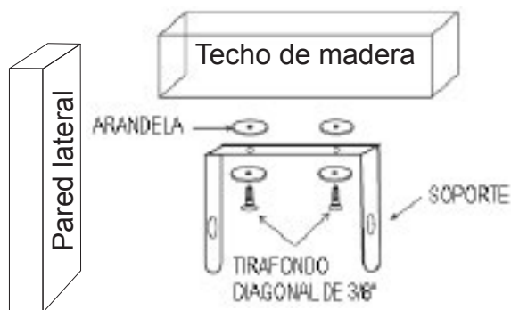
Figura 4b. Montaje de dos tornillos
