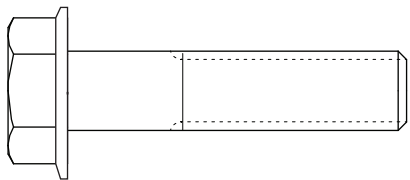
(B) Vis à embase M10 x 25 mm Qté 2
