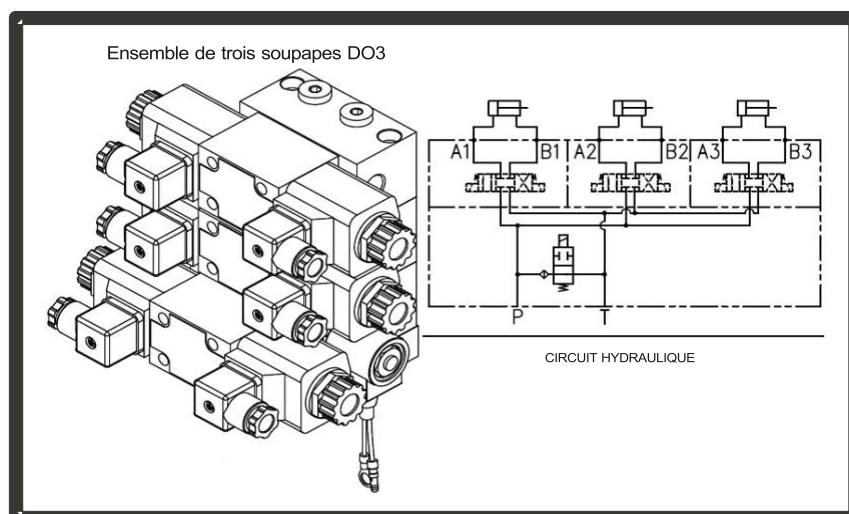
Schéma 3
