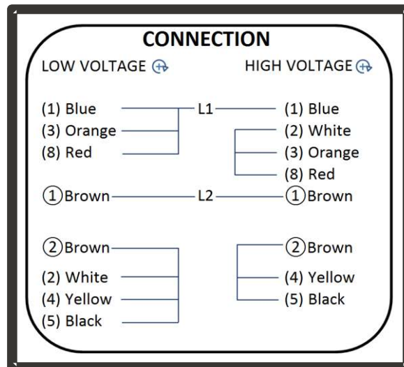
Schéma n° 1
