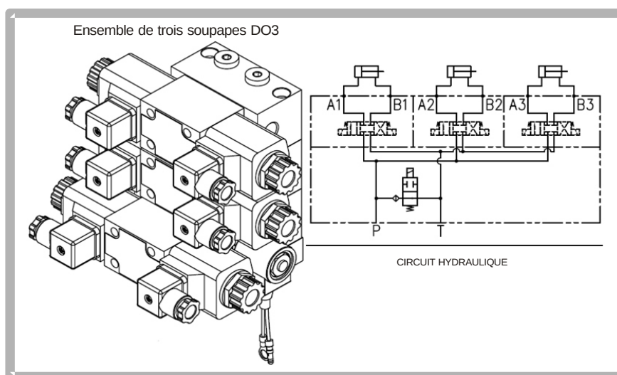
Schéma 3
